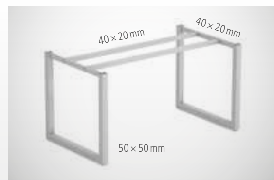
Podnož stolu UNI O (str. 24)
